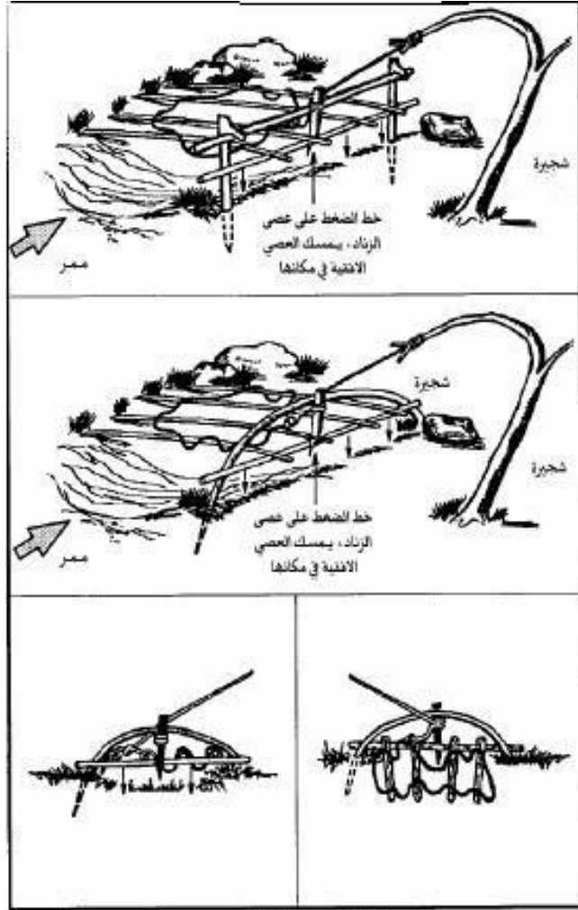
شكل 8 - 11 شرك الدعامة
