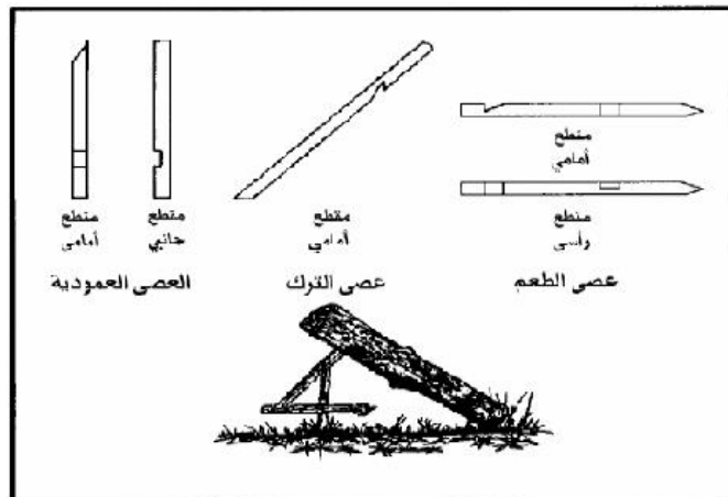
شكل 8 - 12 مصيدة رقم 4
