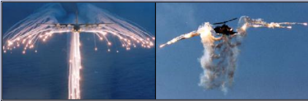
رسم 12. مروحية هجومية كوبرا تطلق قنابل مضيفة ذات حرارة عالية تحاول خداع وإبعاد صواريخ أرض - جو وصواريخ جو-جو التي تلاحق المصدر الحراري (يمين). طائرة شحن عسكري تحاول إبعاد صاروخ موجه حرارياً (يسار)
