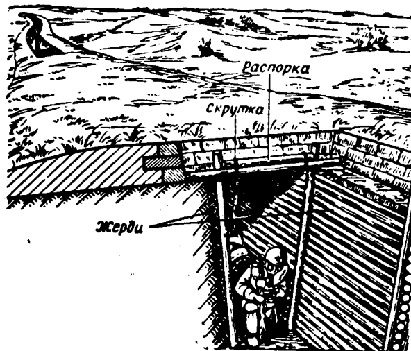
Рис. 4. Перекрытый участок траншеи с крутостями, одетыми жердями
