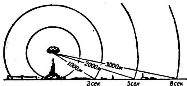
Рис. 3. Скорость распространения ударной волны атомного взрыва
