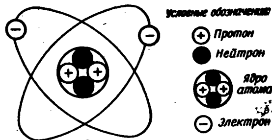
Рис. 1. Схематическое строение атома гелия
