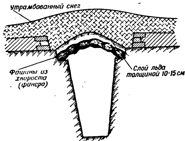
Рис. 5. Перекрытие траншеи или окопа, сделанное из снега
