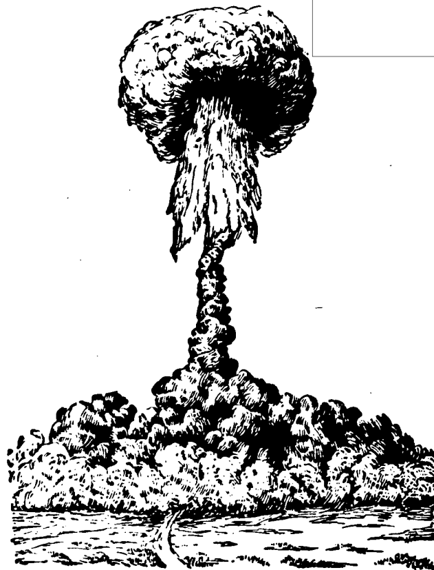
Рис. 2. Грибовидное облако, образующееся при атомном взрыве
