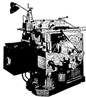
Querhobelmaschine GH 400
