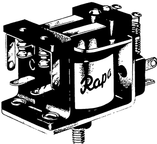
2poliges Gleichstrom-Kleinrelais (ca. 2-fach vergrößert)
