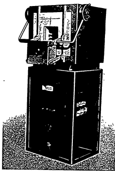
Elektrischer Hochtemperaturofen von maximal 1700° C Ofen-Temperatur
