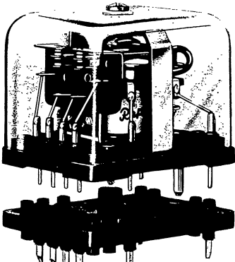
2poliges Steckrelais mit Gehäuse (natürliche Größe)
