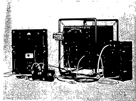
Druckindikator
