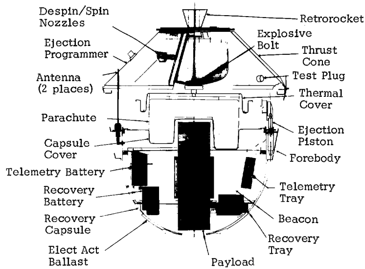
— J-1 System —
