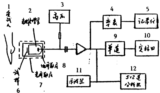
图7: 光子探测系统示意图.
