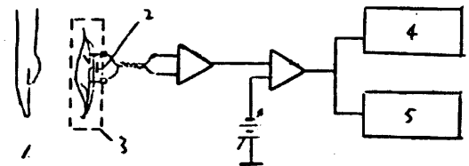
图4: 一种生物探测用显示器示意图, 其中 1. 受试人; 2. 显影; 3. 容器; 4. 示波器; 5. 记录仪
