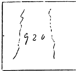
图1: 特异视觉人王××在X光胶片上产生的异常感光投影“920”
