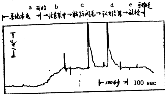
图5: 特异视觉过程的生物探测响应
