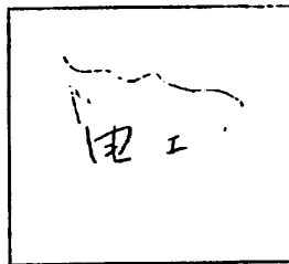
图2: 特异视觉人×××在核乳胶片上产生的异常感光投影“电工”
