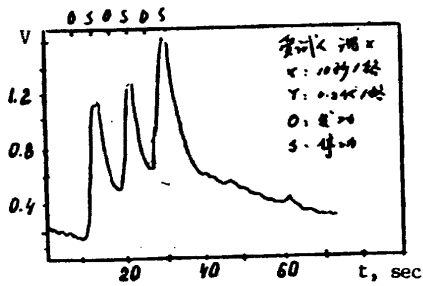
图6: 气功师气的生物探测响应 (沈以作实验)
