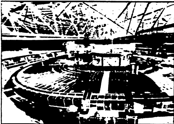
BERKELEY BEVATRON
